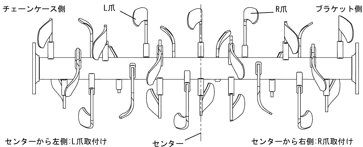
図5 外盛耕全体図（センターから左側にL爪、センターから右側にR爪を組付け）
