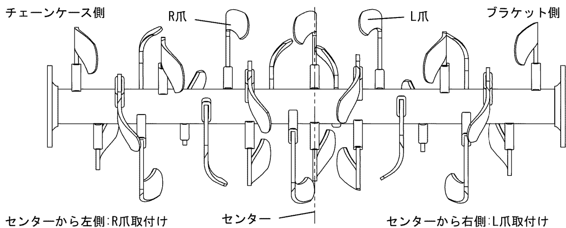
図4 内盛耕全体図（センターから左側にR爪、センターから右側にL爪を組付け）
