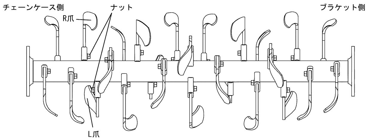
図3 平面耕全体図（爪の曲がり方向にナットがくるように組付け）
