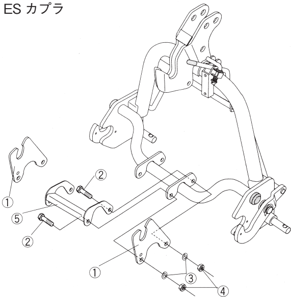
ES カプラ
